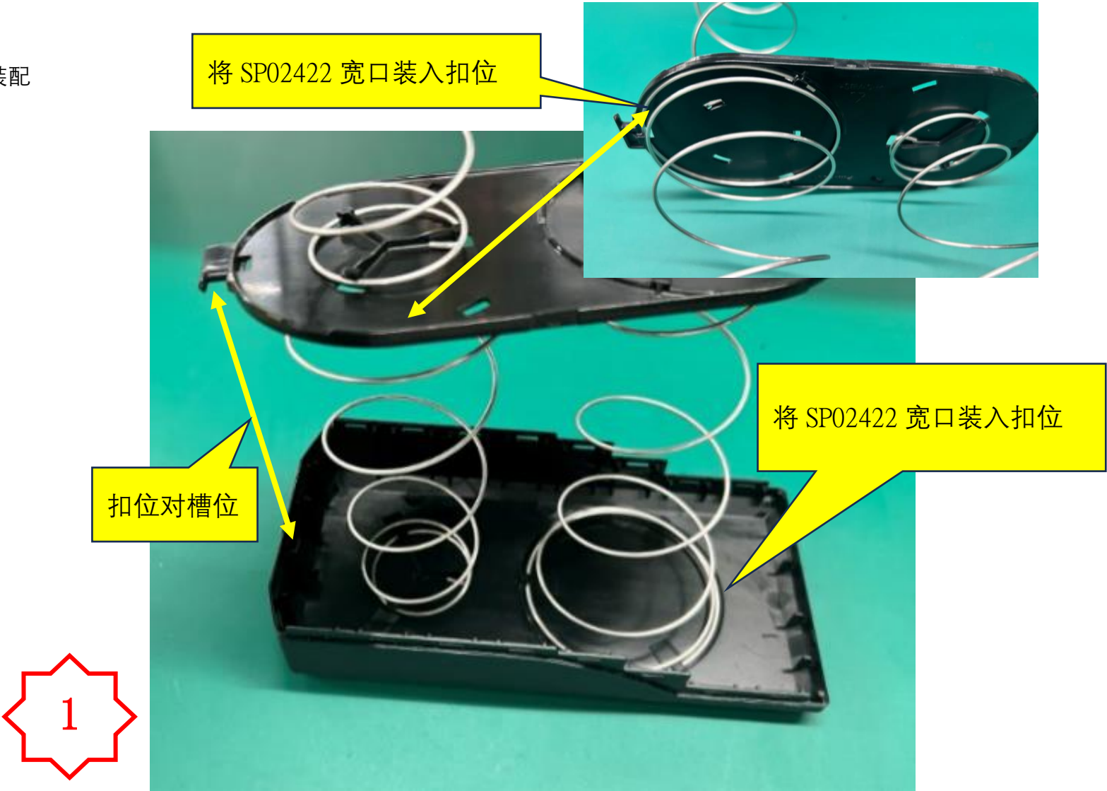
图一，将 PM3578-5 和 PM3578-4 两边未装配的弹簧宽口互装入两个零件的扣位里面，注意装配到位。
