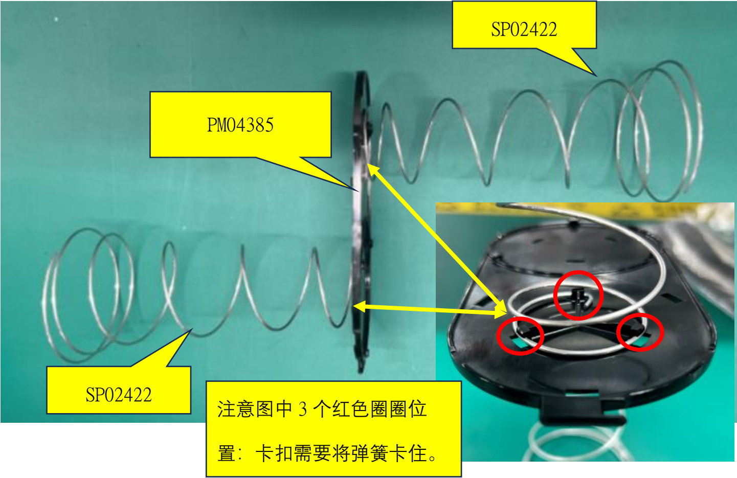
图一，在 PM04385 两边分别装上 SP02422 弹簧，注意 3 个卡扣需扣到位。
