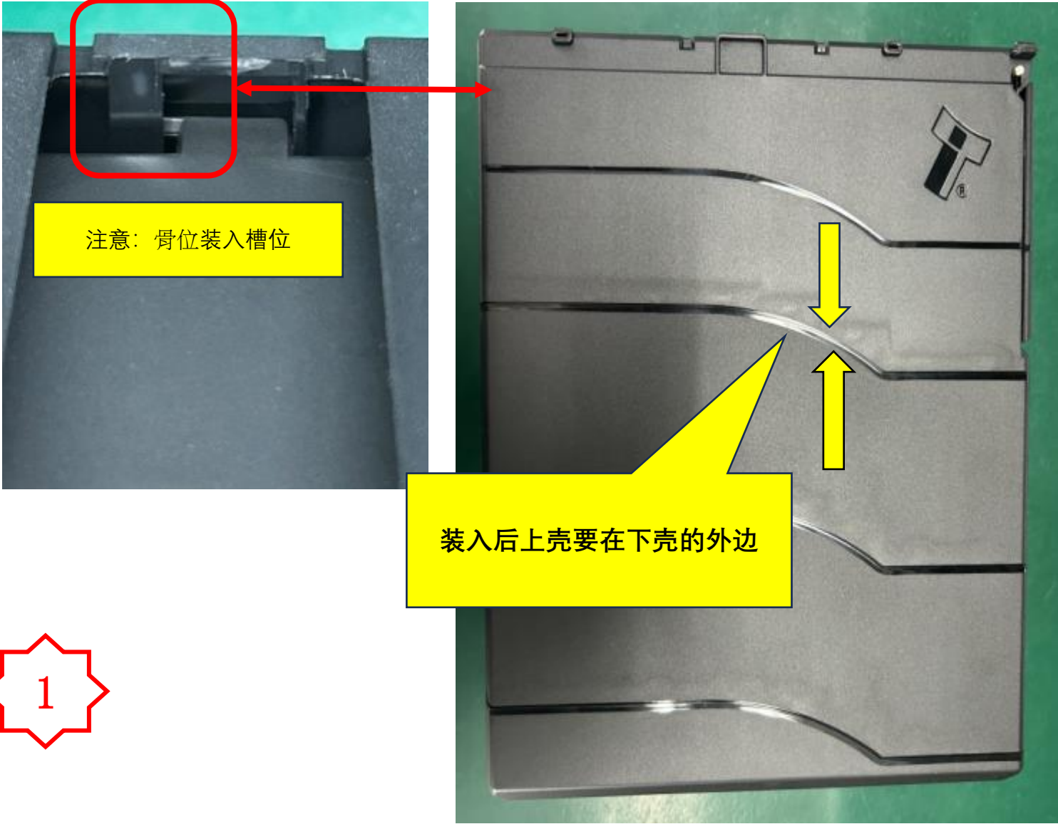
图一，将 PA3578-2 和 PA3578-10 先预装，装入时注意 PM3091 的骨位需装入上壳的槽位，装入后上壳要在下壳的外边，至少要扣入一个以上的卡扣。
