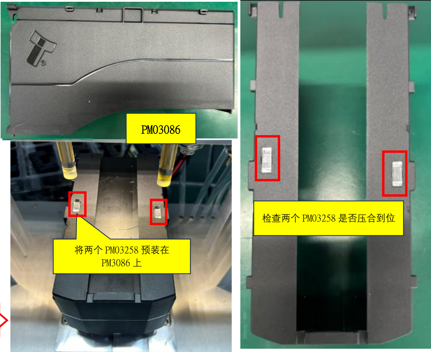
图一，先将 PM03086 放入治具，再将两个 PM3258 分别预装在 PM3086 如图示对应位置，再进行压合，检查两个 PM03258 是否压合到位。
