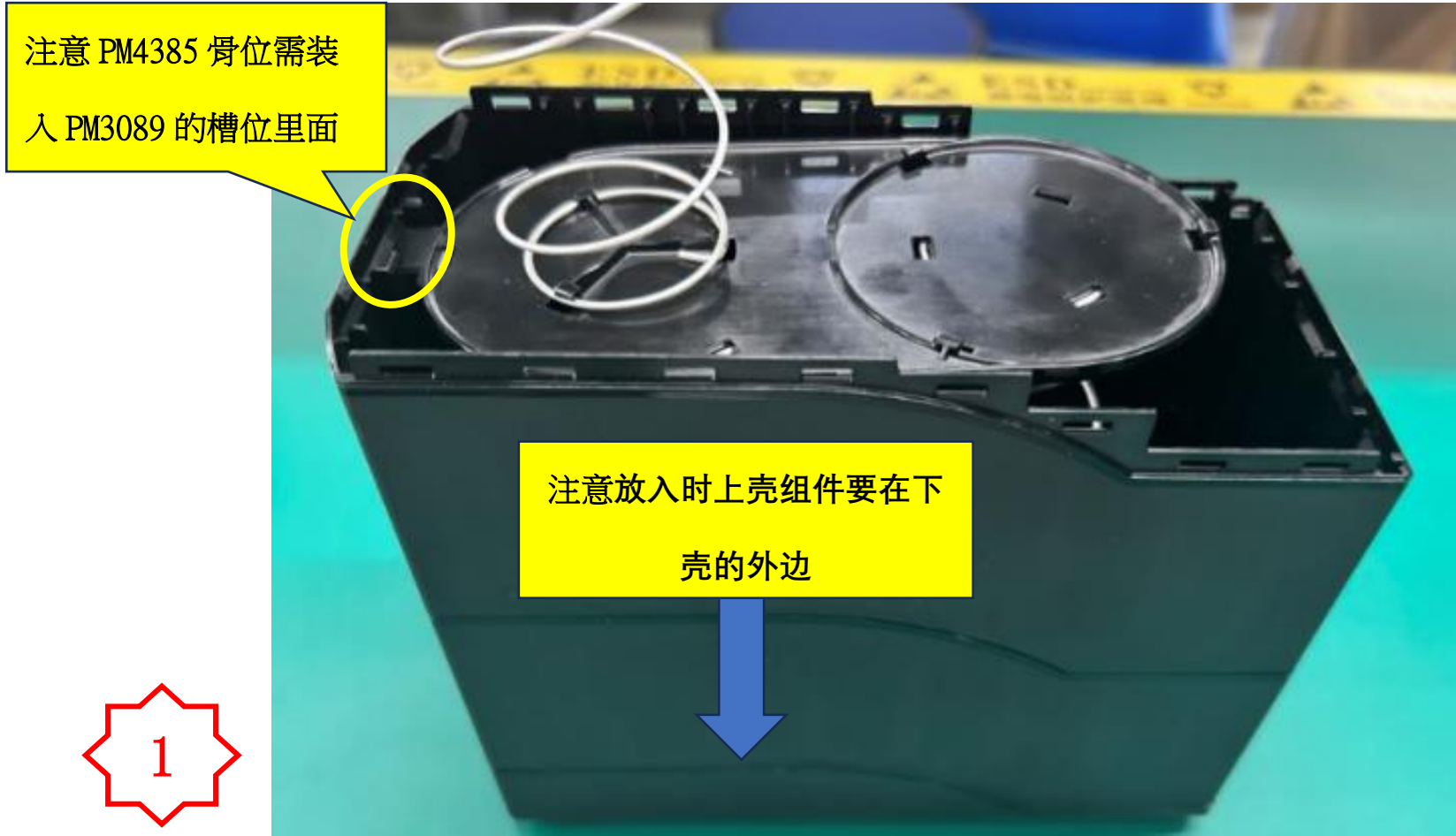
图一，将 PA03578-3 组件装入 PA3578-6 的组件，注意 PM4385 骨位需装入 PM3089 的槽位里面，先将组件预装好，上壳组件要在下壳的外边，至少合上 1 个以上的卡扣。
